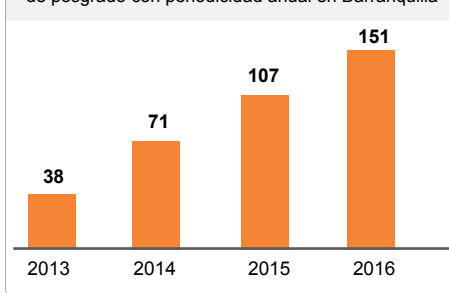
Gráfica 10. Número de matriculados en programas de posgrado con periodicidad anual en Barranquilla
